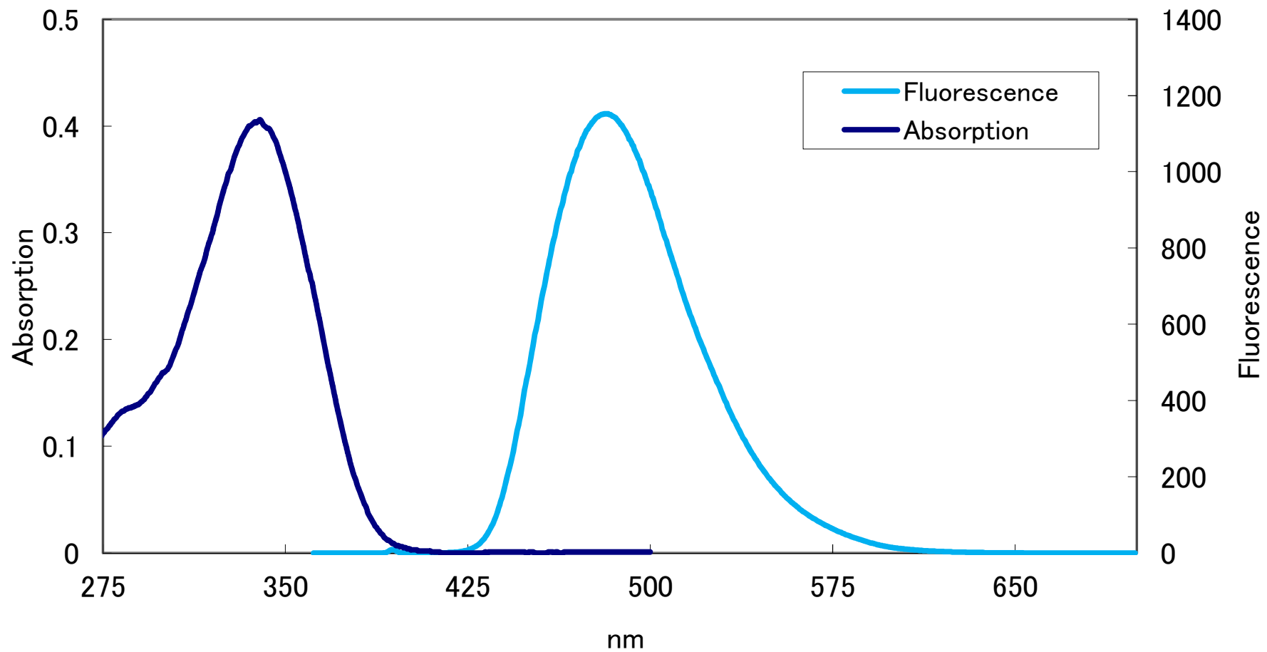
FD-001 吸収発光スペクトル
